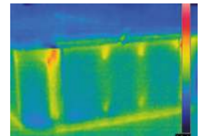
Essai de fuites de chaleur réalisé avec le système Nordic Insulation System
